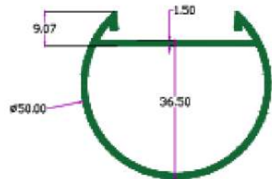
SEC.NO. 4807 Wt. 2.460 TO 2.600 KG./ 12'
