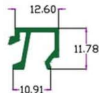
SEC.NO. 4573
