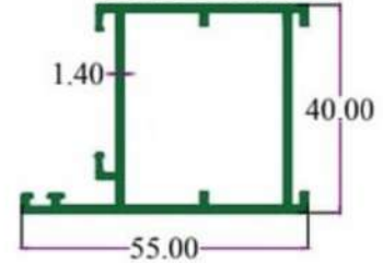
DOOR FRAME
