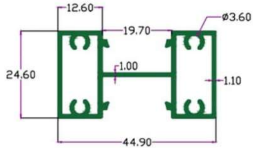
SEC.NO. 4510
