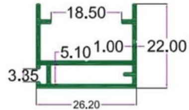
SEC.NO. 4433 WT. 1.000 TO 1.200 KG/12'
