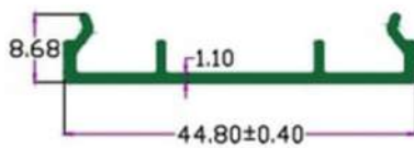
SEC.NO. 4531
