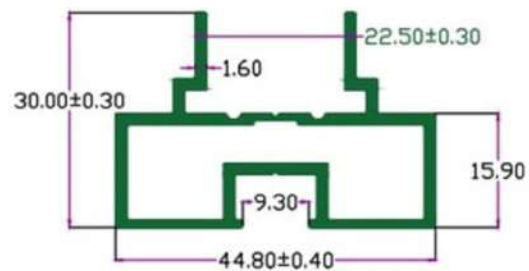
SEC.NO. 4529
