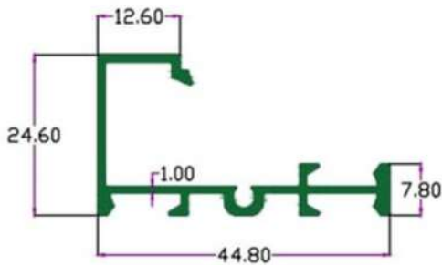
SEC.NO. 4509
