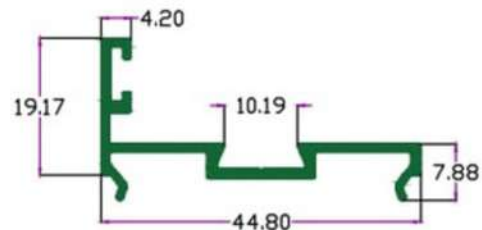
SEC.NO. 4544
