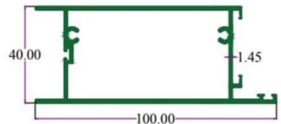
Door Bottom
