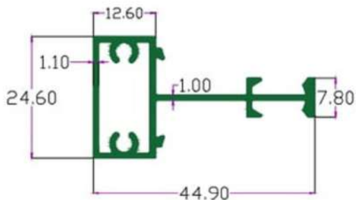
SEC.NO. 4572
