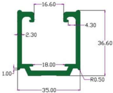
SEC.NO. 4363 Wt. 2.850 TO 3.000 KG./ 12'
