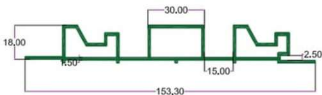
SEC.NO. 4871 WT. 5.380 TO 5.580 KG./ 12'
