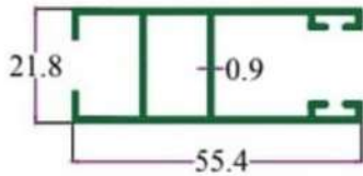
SEC.NO. 3333 WT. 2.800 TO 3.00 KG/ 12'
