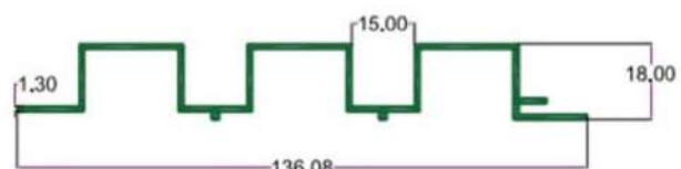
SEC.NO. 4693 WT. 3.100 TO 3.250 KG./ 12'
