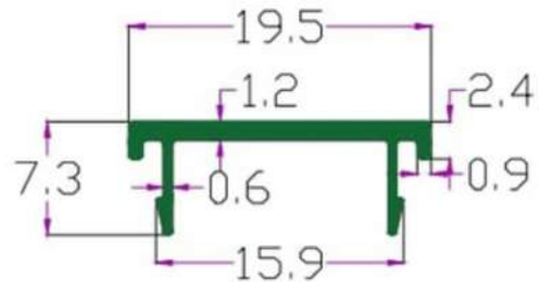
SEC.NO. 4657 Wt. 0.330 TO 0.500 KG./ 12'
