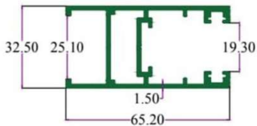
SEC.NO. 4889 WT. 3.700 TO 3.900 KG./ 12'
