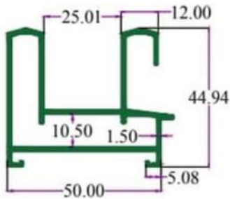
SEC.NO. 4845 WT. 3.650 TO 3.870 KG./ 12'
