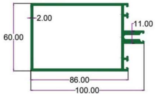
SEC.NO. 4359 WT. 6.500 TO 6.750 KG./ 12'
