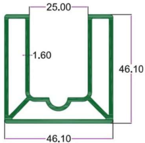
SEC.NO. 4604 WT. 4.400 TO 4.600 KG/12'
