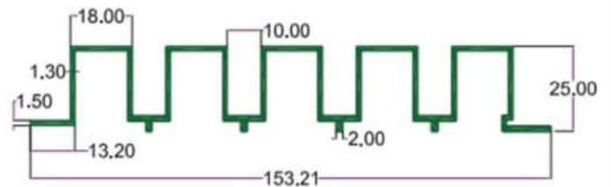
SEC.NO. 4355 WT. 5.130 TO 5.350 KG./ 12'
