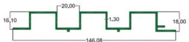
SEC.NO. 4723 WT. 3.220 TO 3.400 KG./ 12'
