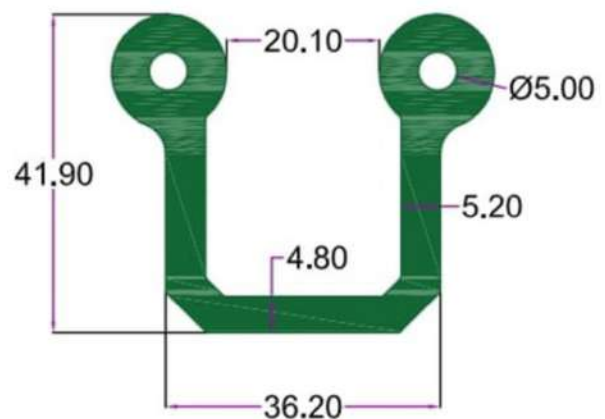
SEC.NO. 4407 WT. 7.000 TO 7.350 KG/12'
