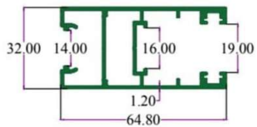
SEC.NO. 4892 WT. 3.360 TO 3.560 KG./ 12'
