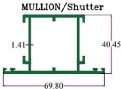
SEC.NO. 3338N WT. 3.300 To 3.500 KG/12'
