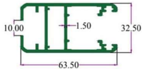
SEC.NO. 3319 WT. 3.850 TO 4.050 KG./12'
