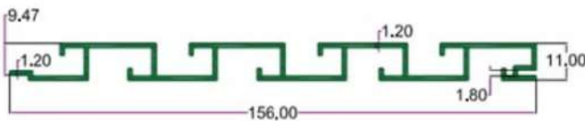
SEC.NO. 4458 WT. 3.750 TO 3.950 KG./ 12'
