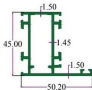
SEC.NO. 4929 WT. 3.225 TO 3.500 KG./ 12'
