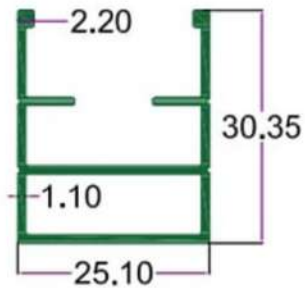
SEC.NO. 4776 WT. 1.290 TO 1.400 KG./ 12'
