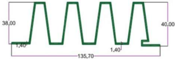
SEC.NO. 4550 WT. 5.660 TO 5.850 KG./ 12'
