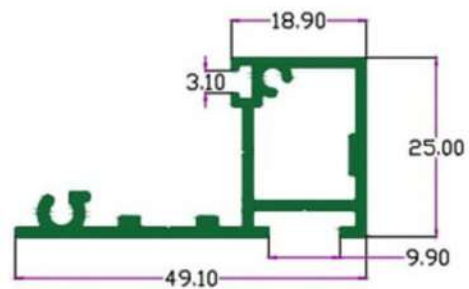
SEC.NO. 4467 Wt. 9.160 TO 9.350 KG./ 12'
