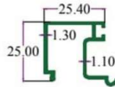
SEC.NO. 4931 WT. 1.200 TO 1.350 KG./ 12'
