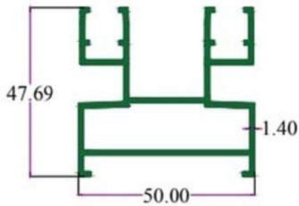
SEC.NO. 4928 WT. 3.600 TO 3.900 KG./ 12'
