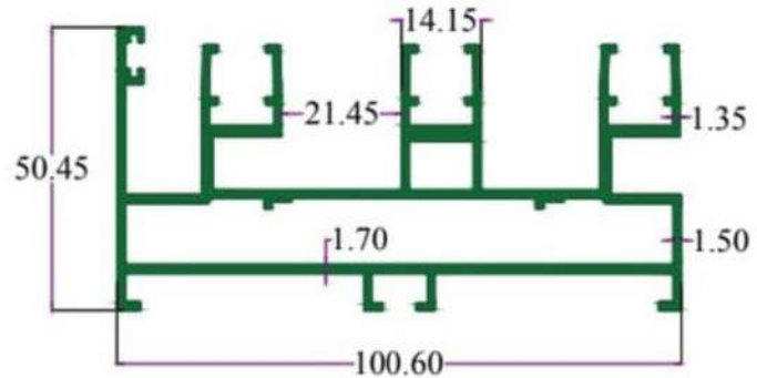
SEC.NO. 4927 WT. 7.615 TO 7.915 KG./ 12'
