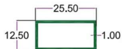
SEC.NO. 4779 WT. 0.700 TO 0.800 KG./ 12'
