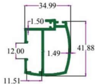
SEC.NO. 4843 WT. 4.180 TO 4.400 KG./ 12'
