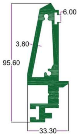
SEC.NO. 4274 WT. 10.050 TO 10.500 KG/12'
