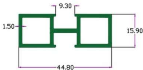
SEC.NO. 4685 Wt. 2.000 TO 2.200 KG./ 12'
