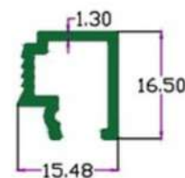
SEC.NO. 4716 Wt. 0.700 TO 0.820 KG./ 12'
