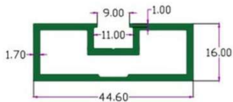
SEC.NO. 4429(K.I) Wt. 2.120 TO 2.300 KG./ 12'
