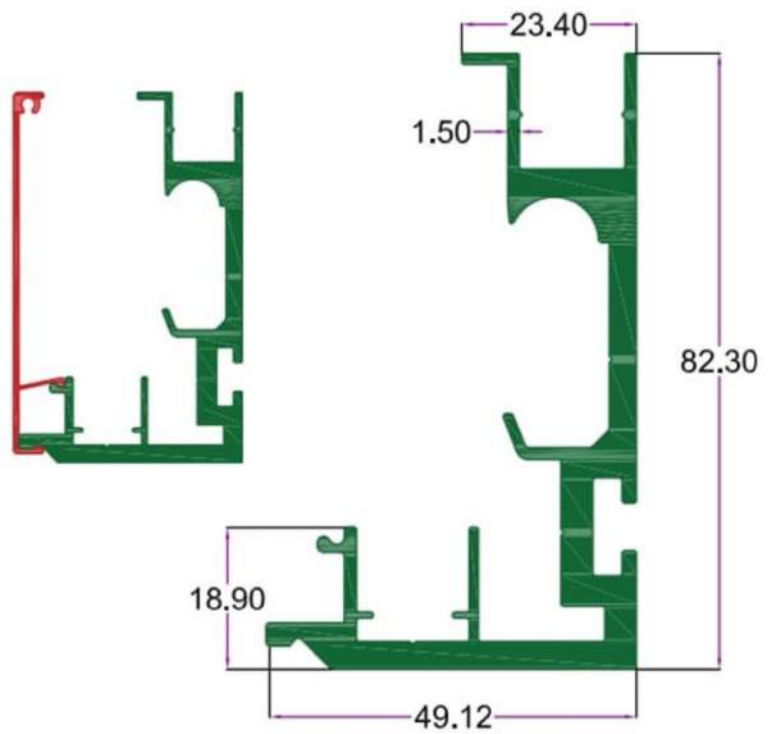
SEC.NO. 4667 WT. 6.800 TO 7.100 KG/12'
