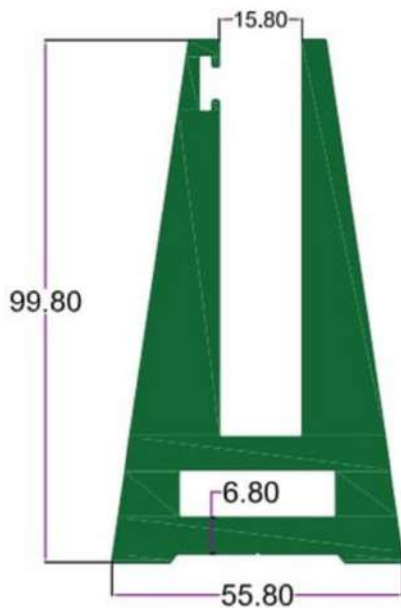
SEC.NO. 5197 WT. 25.000 TO 25.500 KG/12'
