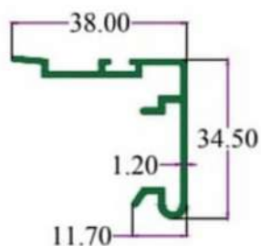
SEC.NO. 4891 WT. 1.230 TO 1.380 KG./ 12'
