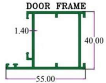
SEC.NO. 3334N WT. 2.650 To 2.850 KG/12'
