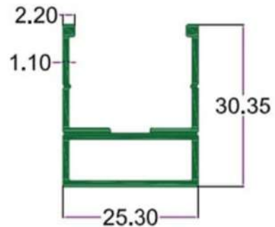
SEC.NO. 4777 WT. 1.340 TO 1.450 KG./ 12'
