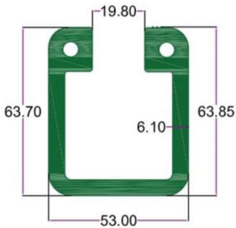
SEC.NO. 4763 WT. 12.500 TO 12.900 KG/12'
