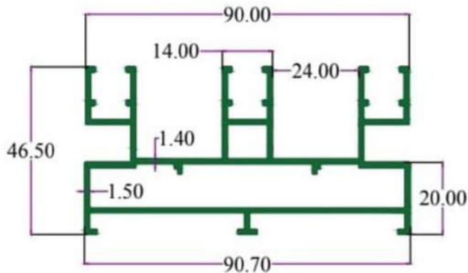
SEC.NO. 4888 WT. 5.900 TO 6.150 KG./ 12'
