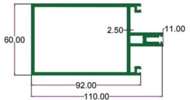
SEC.NO. 4372 WT. 9.270 TO 9.750 KG./ 12'
