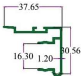
SEC.NO. 4926 WT. 1.310 TO 1.450 KG./ 12'
