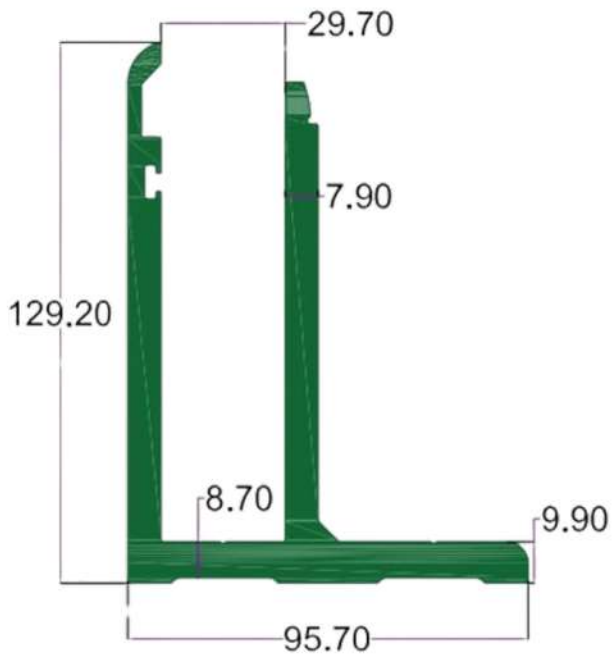
SEC.NO. 4681 WT. 25.300 TO 25.500 KG/12'
