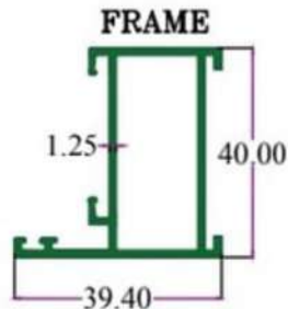
SEC.NO. 3337N WT. 2.000 To 2.200 KG/12'
