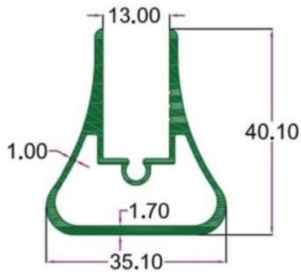
SEC.NO. 4330 WT. 2.200 TO 2.400 KG/12'
