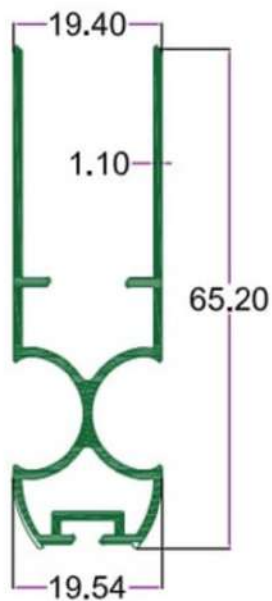
SEC.NO. 4778 WT. 2.000 TO 2.150 KG./ 12'
