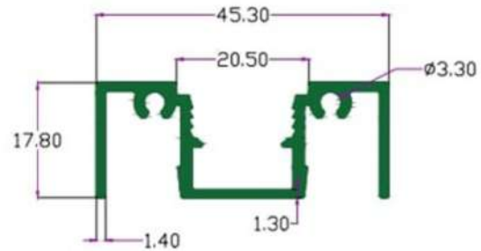
SEC.NO. 4691 Wt. 1.830 TO 2.050 KG./ 12'
