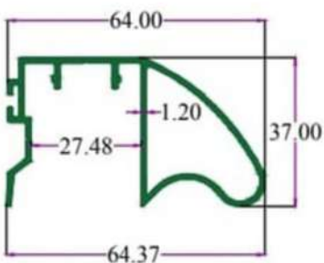
SEC.NO. 4847 WT. 2.580 TO 2.850 KG./ 12'
