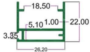
SEC.NO. 4433 WT. 1.000 TO 1.200 KG/12'
