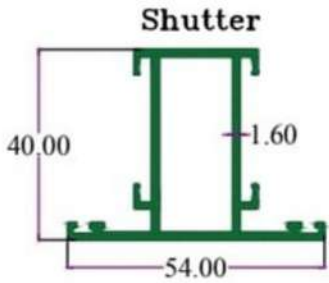
SEC.NO. 3332N / 4766 WT. 2.800 To 3.000 KG/12'
