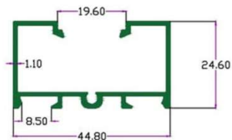
SEC.NO. 4508 Wt. 1.580 TO 1.700 KG./ 12'
