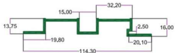
SEC.NO. 4291 WT. 3.350 TO 3.600 KG./ 12'
