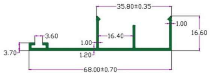
SEC.NO. 4366 Wt. 1.300 TO 1.450 KG./ 12'
