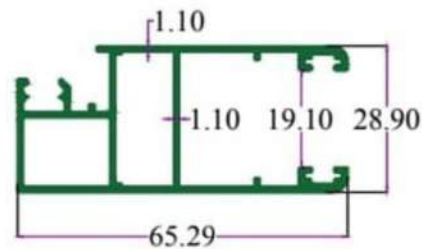
SEC.NO. 4925 WT. 2.750 TO 3.050 KG./ 12'
