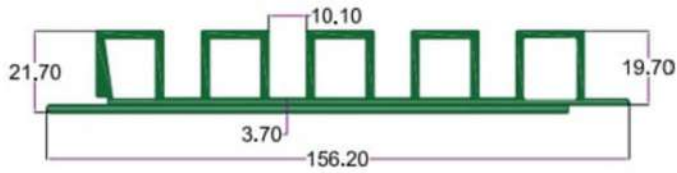
SEC. NO. 4097 WT. 10.100 TO 10.500 KG./12'
