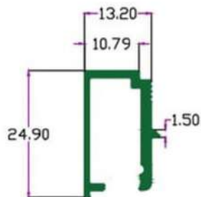
SEC.NO. 4468 Wt. 0.860 TO 0.100 KG./ 12'
