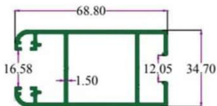
SEC.NO. 4842 WT. 3.760 TO 4.000 KG./ 12'
