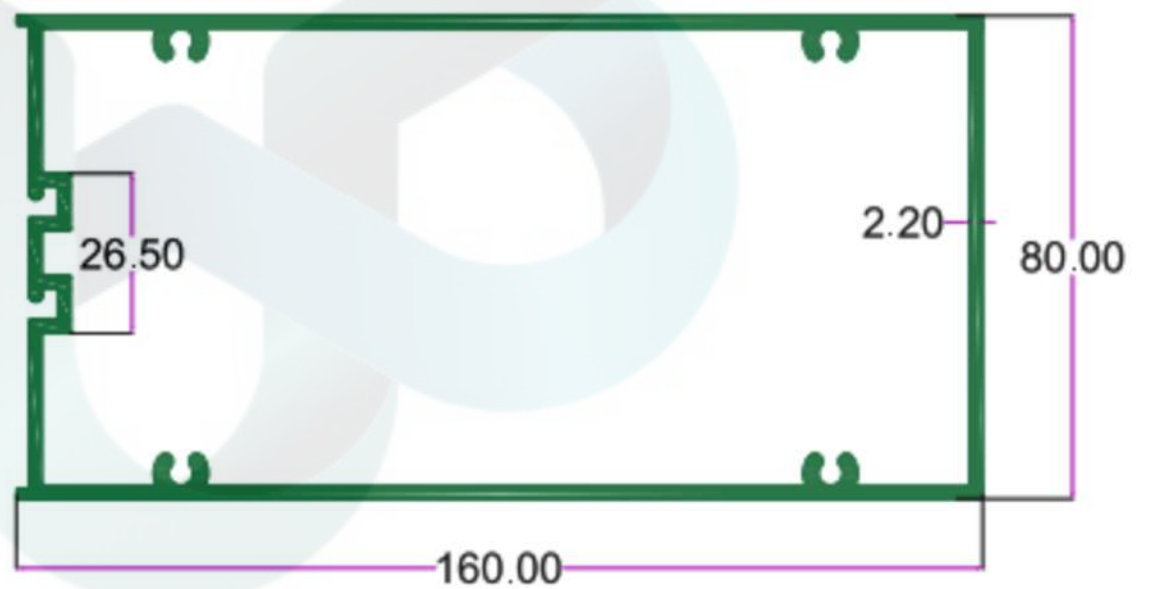
SEC.NO. 4987 WT. 11.770 TO 12.400 KG/12'
