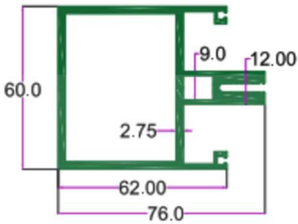
SEC. No. 2439 WT. 8.000 TO 8.500 KG/I2'
