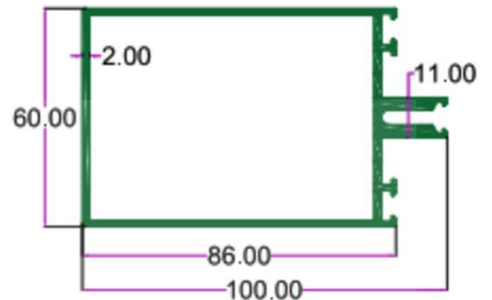
SEC.NO. 4359 WT. 6.500 TO 6.750 KG/I2'
