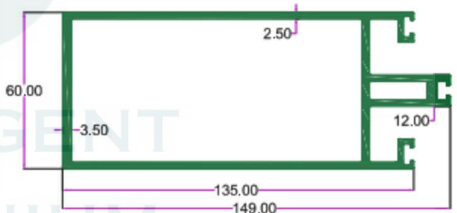
SEC.NO. 5361 WT. 12.570 TO 12.780 KG/I2'
