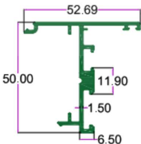
SEC.NO. 4804 WT. 2.380 TO 2.600 KG/12'
