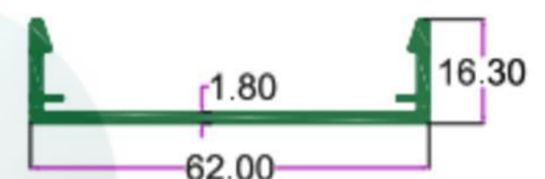
SEC.NO. 4480 WT. 1.730 TO 2.000 KG/12'
