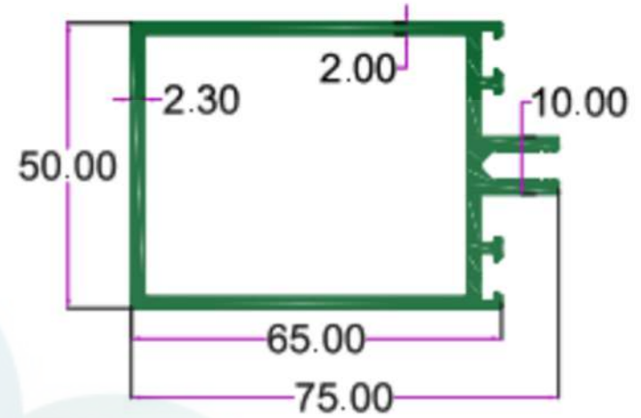
SEC.NO. 4864 WT. 5.500 TO 5.750 KG./ 12'
