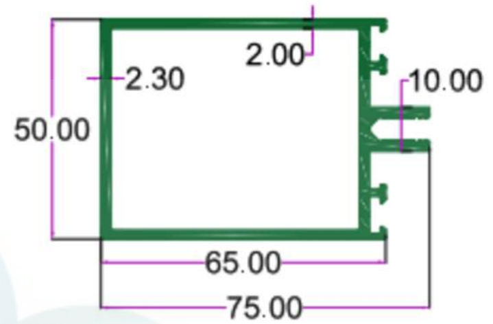
SEC.NO. 4864 WT. 5.500 TO 5.750 KG./ 12'
