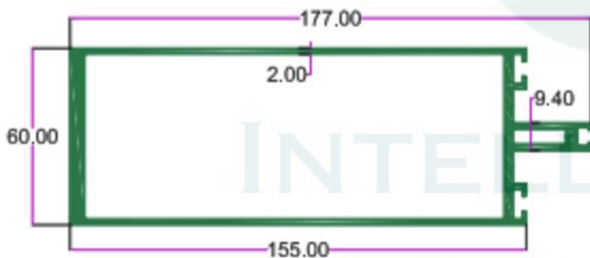
SEC.NO. 5212 WT. 12.190 TO 12.610 KG/I2'
