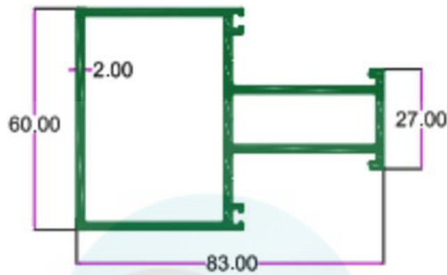
SEC.NO. 4859 WT. 6.200 TO 6.450 KG/I2'
