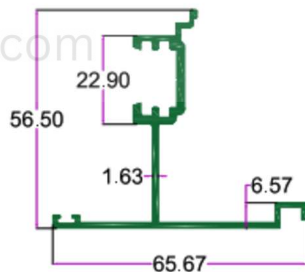
SEC.NO. 4803 WT. 2.610 TO 2.850 KG/12'
