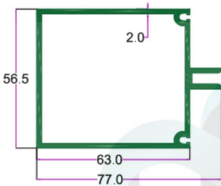
SEC. NO. 2436 WT. 7.000 TO 7.500 KG./15'
