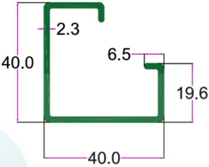
SEC.No. 2044 WT. 2.600 TO 2.800 KG/12'
