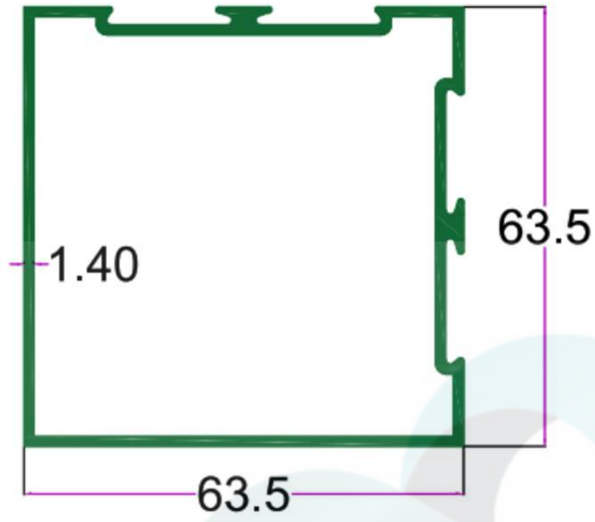
SEC.No. 1757 WT. 4.00 TO 5.00 KG/15'
