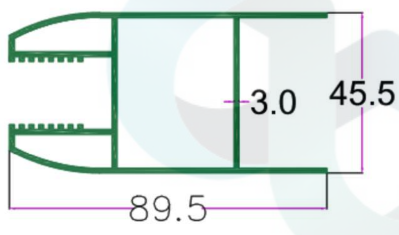
SEC.No. 1759 WT. 8.500 TO 9.500 KG/15'
