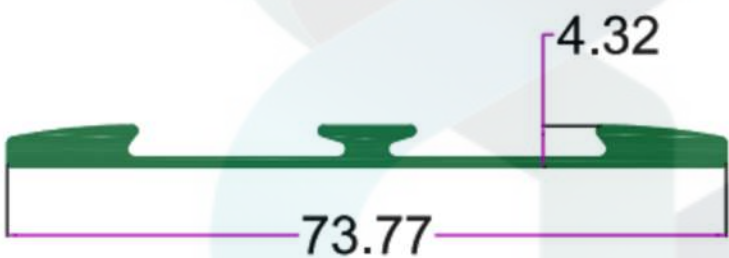
SEC.NO. 3317 WT. 2.000 TO 2.500 KG/12'
