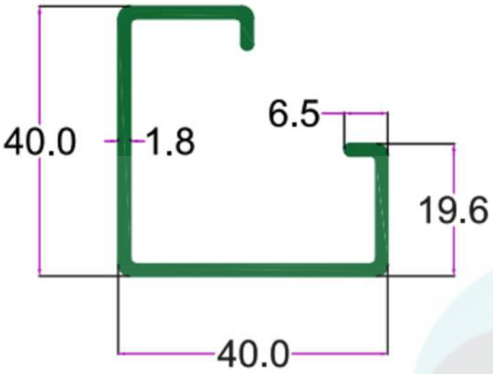
SEC.No. 2043 WT. 2.100 TO 2.300 KG/12'
