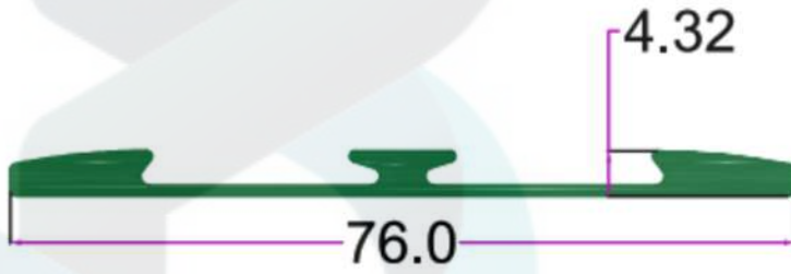
SEC.NO. 3318 WT. 2.200 TO 2.600 KG/12'
