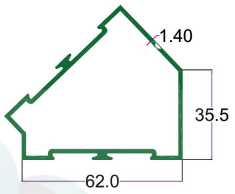
SEC.No. 1756 WT. 3.800 TO 5.00 KG/15'
