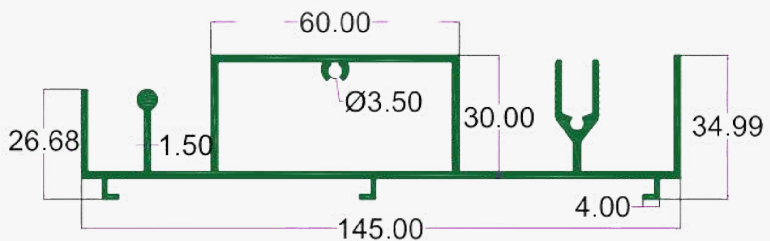
SEC.NO. 4581 WT. 6.730 TO 6.900 KG/12'
