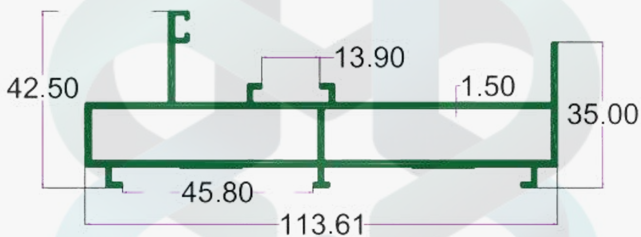
SEC.NO. 4580 WT. 5.140 TO 5.300 KG/12'
