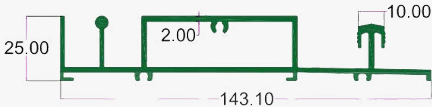
SEC.NO. 4582 WT. 6.280 TO 6.400 KG/12'
