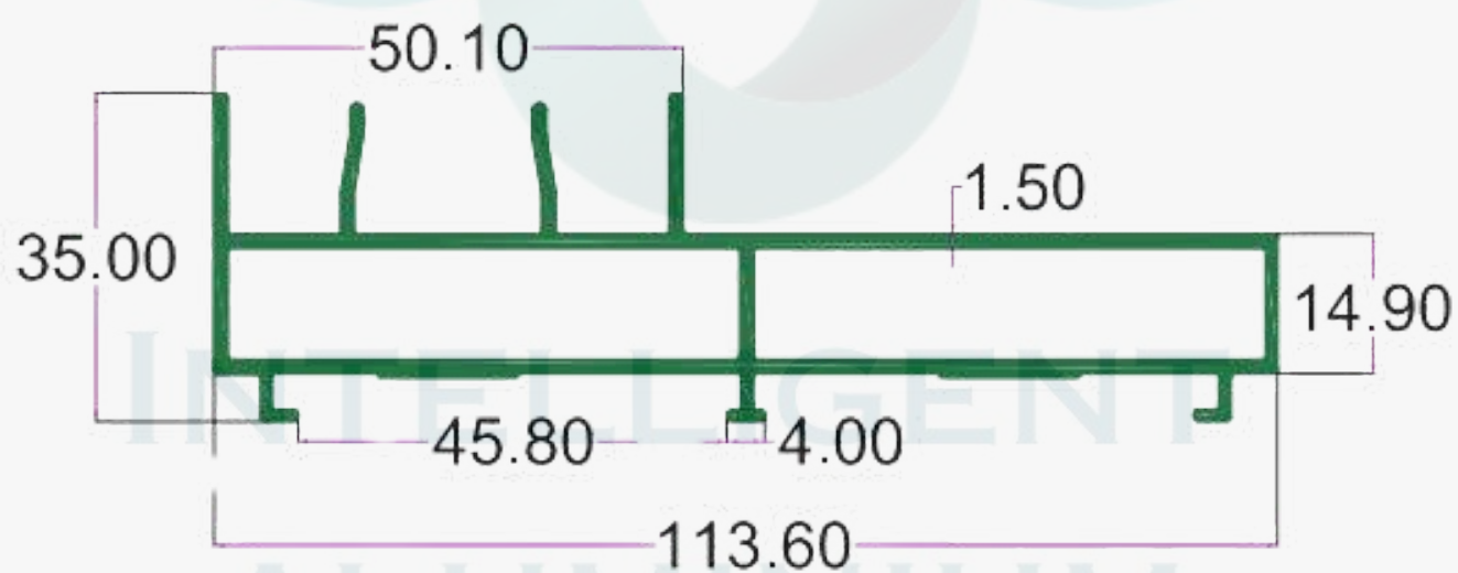
SEC.NO. 4579 WT. 5.140 TO 5.300 KG/12'
