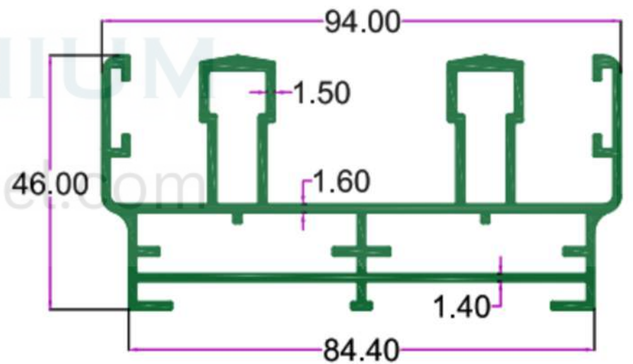
SEC.NO. 4345 WT. 7.100 TO 7.300 KG./ 12'
