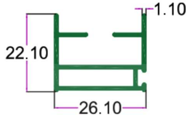
SEC.NO. 5106 WT. 1.130 TO 1.380 KG/12'
