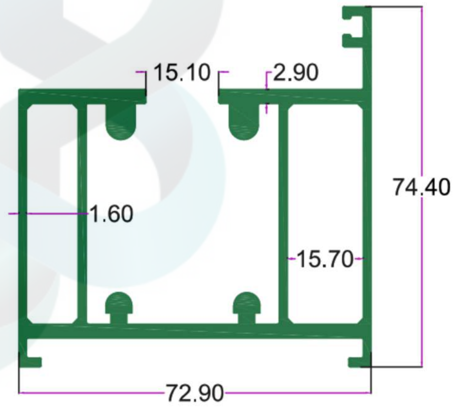
SEC.NO. 5008 WT. 8.860 TO 9.300 KG/I2'
