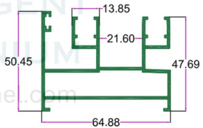
SEC.NO. 5152 WT. 4.600 TO 4.800 KG/12'
