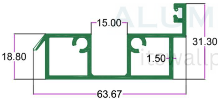
SEC.NO. 5010 WT. 2.900 TO 3.150 KG/I2'
