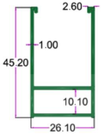
SEC.NO. 4431 WT. 1.400 TO 1.600 KG/12'
