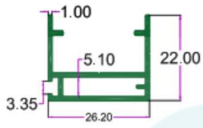
SEC.NO. 4433 WT. 1.000 TO 1.200 KG/12'
