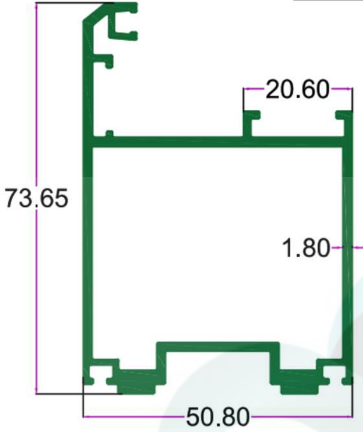
SEC.NO. 5006 WT. 4.735 TO 4.950 KG/12'
