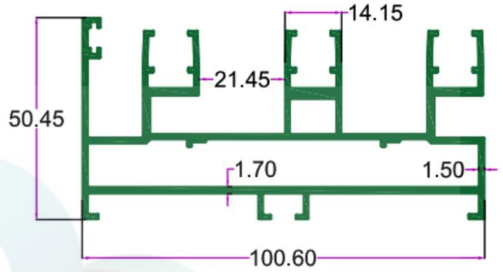
SEC.NO. 4927 WT. 7.615 TO 7.915 KG./ 12'
