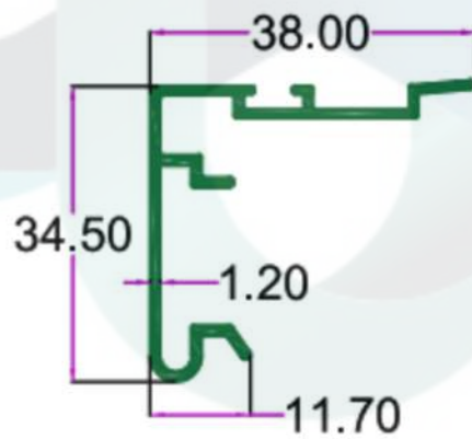
SEC.NO. 4891 WT. 1.230 TO 1.380 KG/12'
