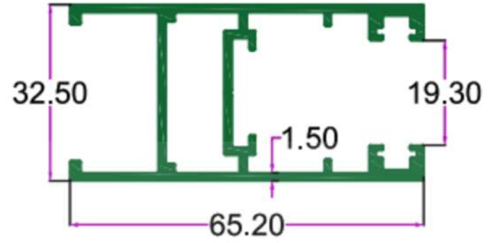
SEC.NO. 4889 WT. 3.700 TO 3.900 KG./ 12'
