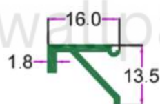
SEC.NO. 3335 WT. 2.500 TO 2.700 KG/12'
