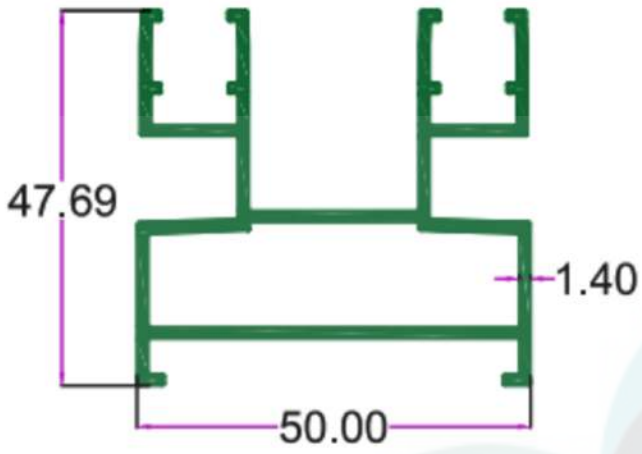
SEC.NO. 4928 WT. 3.600 TO 3.900 KG./ 12'
