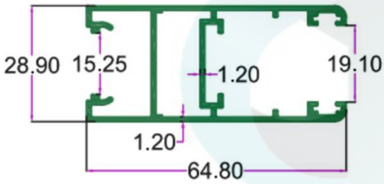
SEC.NO. 4924 WT. 2.990 TO 3.300 KG/12'
