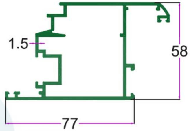
SEC.NO. 4774 WT. 5.150 TO 5.400 KG/I2'
