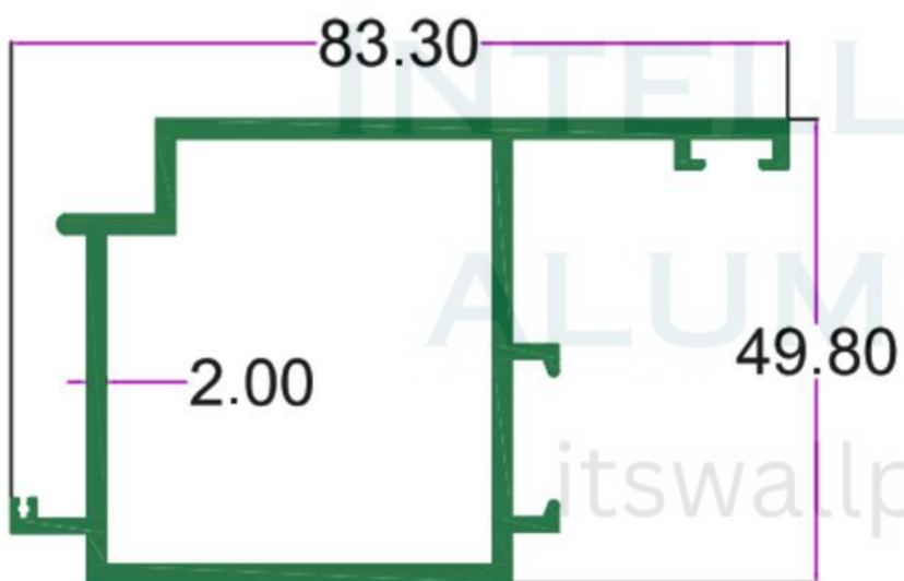
SEC. NO. 3933 WT. 4.700 TO 5.000 KG/I2'
