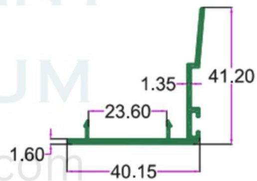
SEC.NO. 4997 WT. 1.375 TO 1.500 KG/12'
