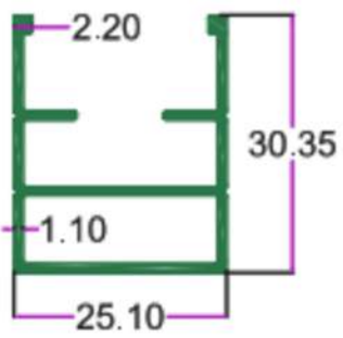
SEC.NO. 4776 WT. 1.290 TO 1.400 KG/12'
