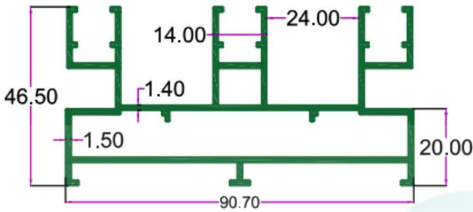
SEC.NO. 4888 WT. 5.900 TO 6.150 KG./ 12'
